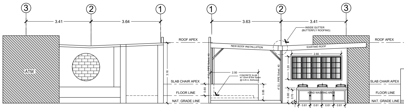
L. SIDE ELEVATION SCALE : 1 : 100 m
